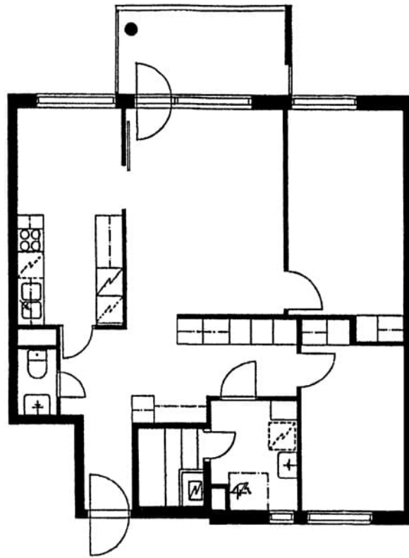
Kyyhkysmäki 7 B 17 / pohjakuva Ei mittakaavassa
