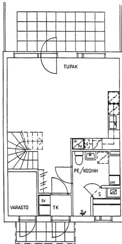
Viestitie 29 E 5 / pohjakuva 1. kerros Ei mittakaavassa
