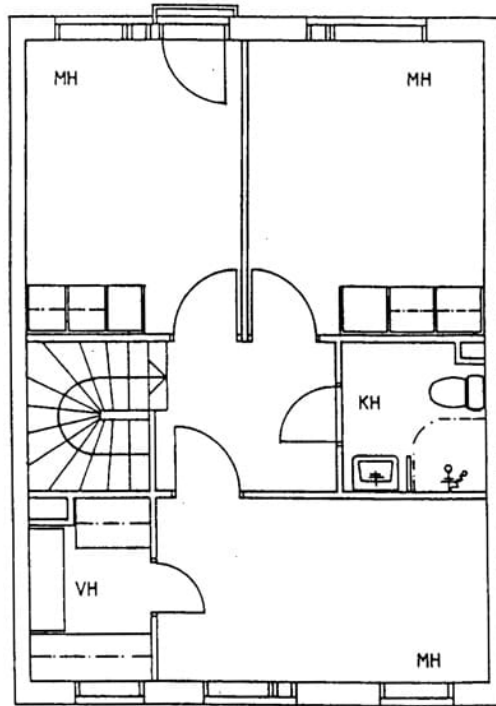
Viestitie 29 E 5 / pohjakuva 2. kerros Ei mittakaavassa
