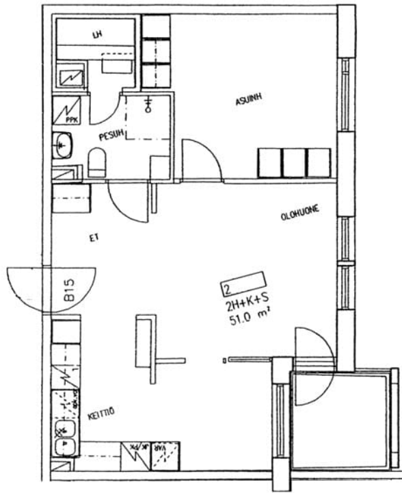
Kangastuvankatu 3 A 13 / pohjakuva Ei mittakaavassa
