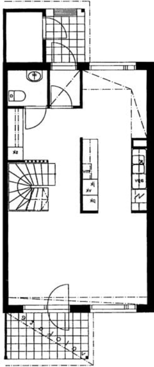
Vasamakatu 5-7 B 19 / pohjakuva 1. kerros Ei mittakaavassa
