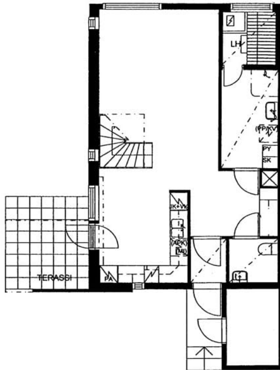
Ruutikuja 5 D 18 / pohjakuva 1.kerros Ei mittakaavassa
