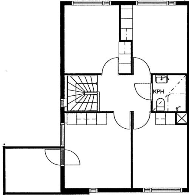
Ruutikuja 5 D 18 / pohjakuva 2.kerros Ei mittakaavassa
