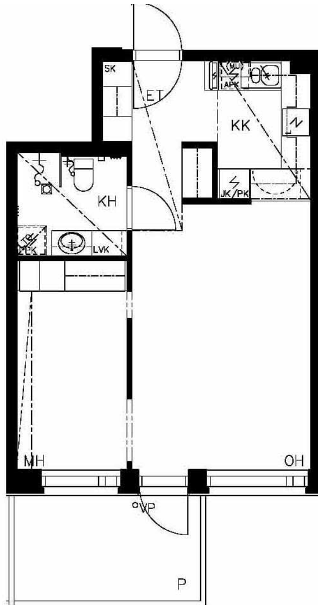
Piilipuuntie 3 D 65 / Pohjakuva Ei mittakaavassa
