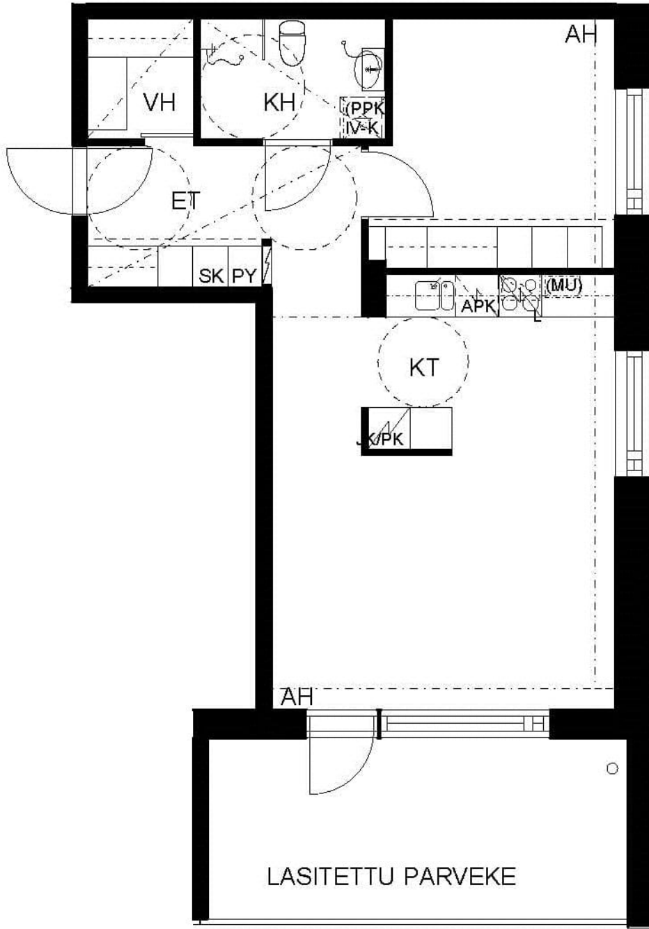
Ulrikankuja 18 B 20 / pohjakuva Ei mittakaavassa
