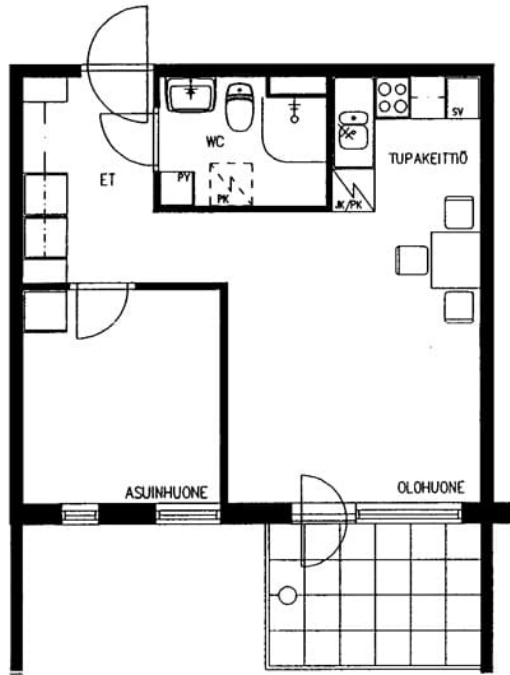
Hovinkatu 5 D 40 / pohjakuva Ei mittakaavassa
