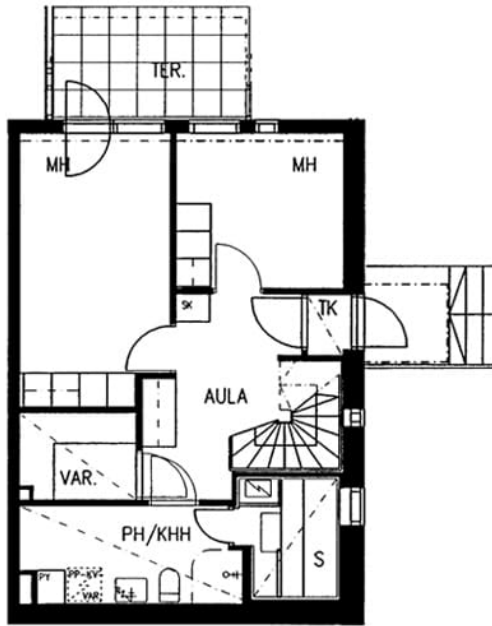
Sienitie 47 C 5 / pohjakuva 1. kerros Ei mittakaavassa
