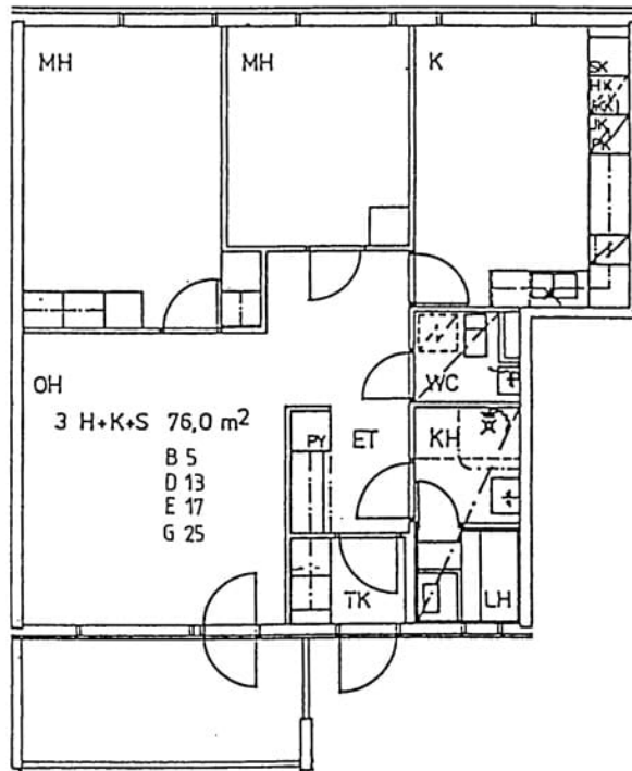
Kääntökuja 3 G 25 / pohjakuva Ei mittakaavassa
