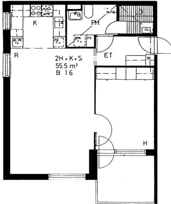
Iso-Hollonkuja 8 B 20 / pohjakuva Ei mittakaavassa
