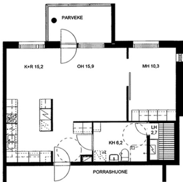
Hukkasenkuj 1 A 10 / pohjakuva Ei mittakaavassa
