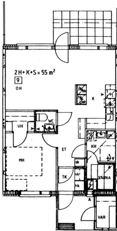
Kihmulantie 4 B 9 / pohjakuva Ei mittakaavassa
