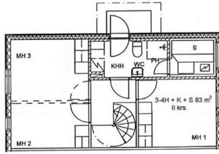
Pullerikinahde 2 B 4 / Pohjakuva Ei mittakaavassa
