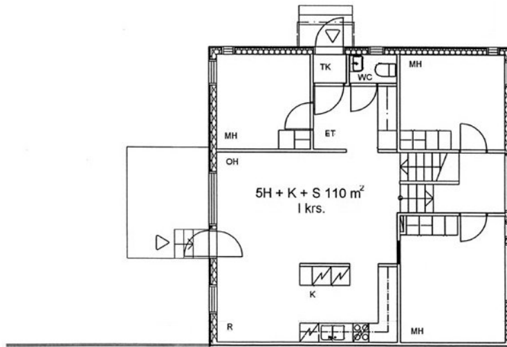
Pullerikinahde 6 D 9 / Pohjakuva Ei mittakaavassa
