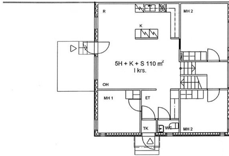
Pullerikinahde 4 I 18 / Pohjakuva Ei mittakaavassa
