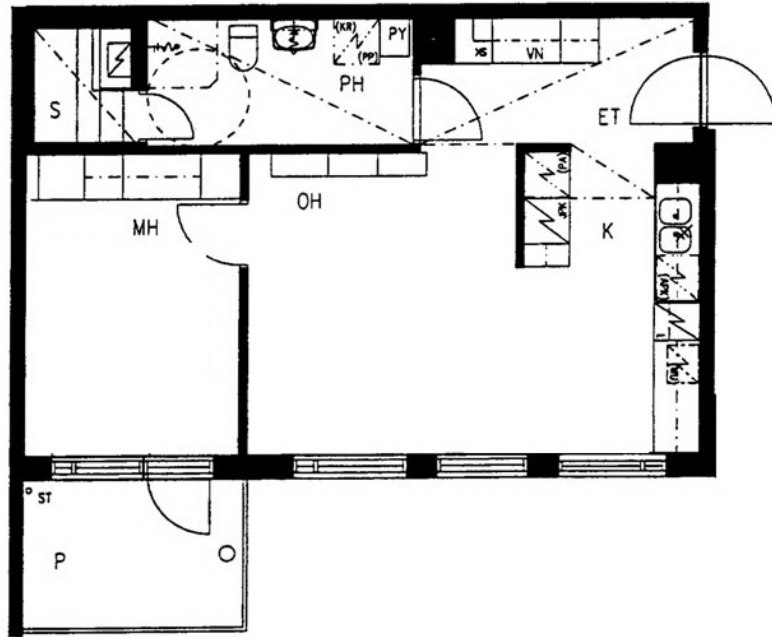
Suurspääntie 9 A 1 / Pohjakuva Ei mittakaavassa
