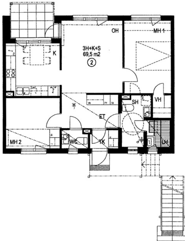
Sepontie 2 A 2 / pohjakuva Ei mittakaavassa
