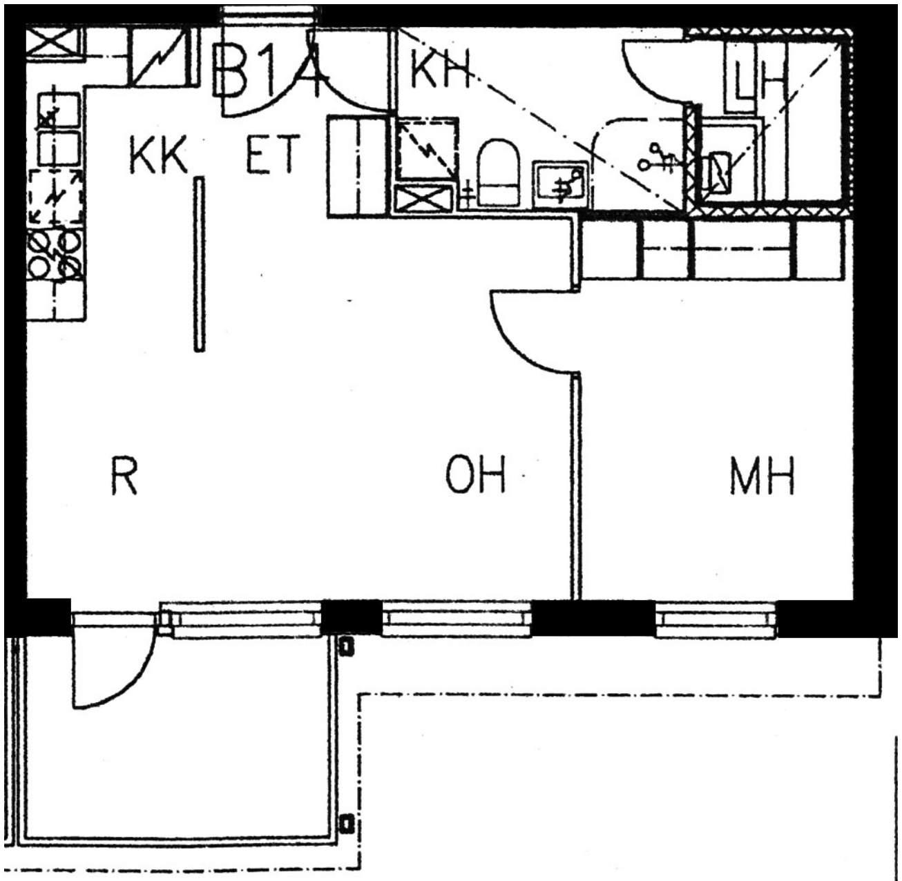
Vahtokuja 2 B 14 / Pohjakuva Ei mittakaavassa
