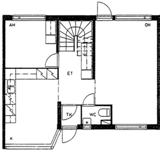
Tapani Löfvinginkatu 2 C 15 / pohjakuva 1. kerros Ei mittakaavassa
