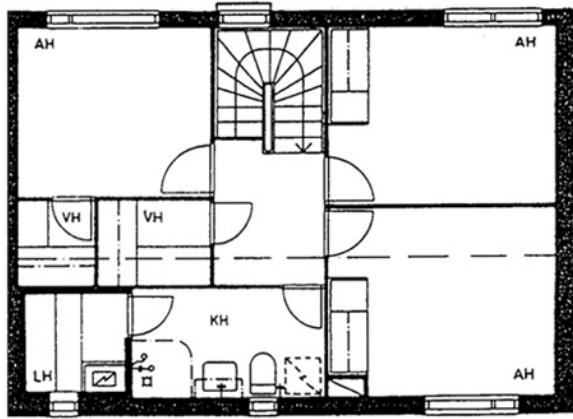
Tapani Löfvinginkatu 2 C 15 / pohjakuva 2. kerros Not in scale
