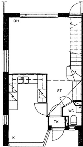
Tapani Löfvinginkatu 2 B 5 / pohjakuva 1. kerros Ei mittakaavassa
