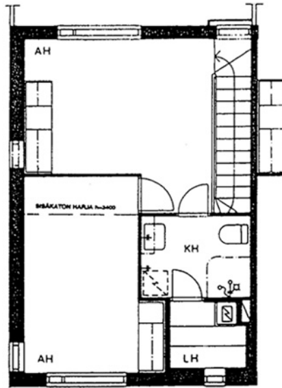
Tapani Löfvinginkatu 2 B 5 / pohjakuva 2. kerros Ei mittakaavassa
