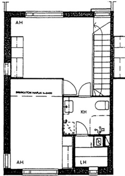
Tapani Löfvinginkatu 2 A 1 / pohjakuva 2. kerros Ei mittakaavassa
