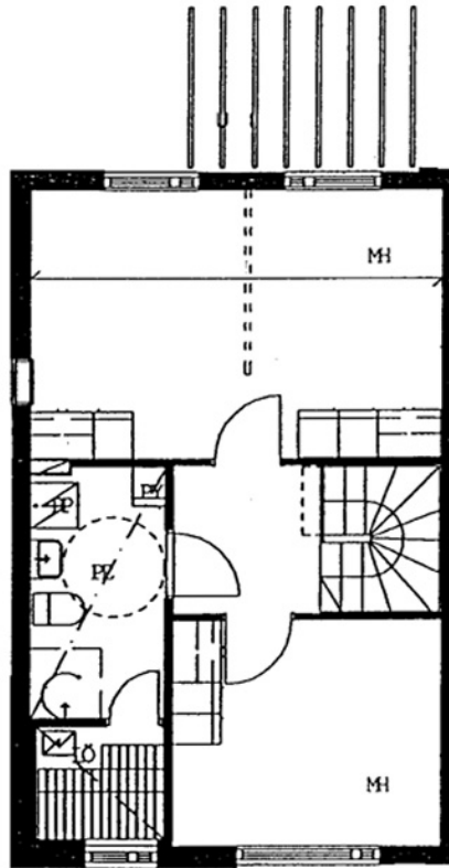
Lehtimäenkuja 4 B 5 / pohjakuva 2. kerros Ei mittakaavassa
