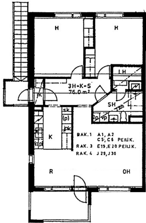
Saagate 10 A 2 / pohjakuva Ei mittakaavassa
