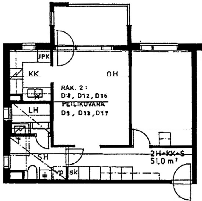
Saagatie 10 D 8 / pohjakuva Ei mittakaavassa
