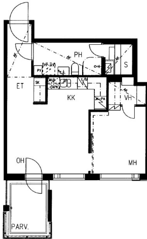
Trillakatu 3 C 40 / pohjakuva Ei mittakaavassa
