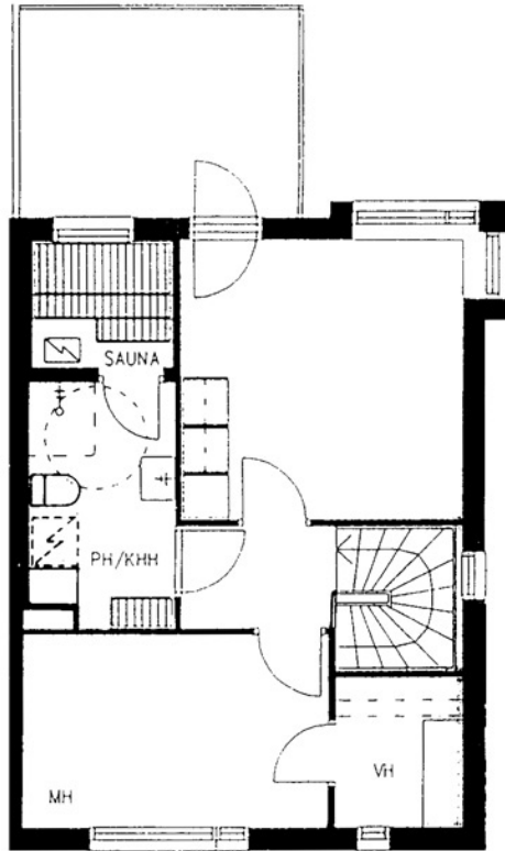
Uudisraivaajankuja 1 C 2 / pohjakuva 2. kerros Ei mittakaavassa
