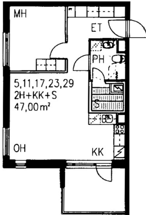
Taapelikatu 6 A 23 / pohjakuva Ei mittakaavassa
