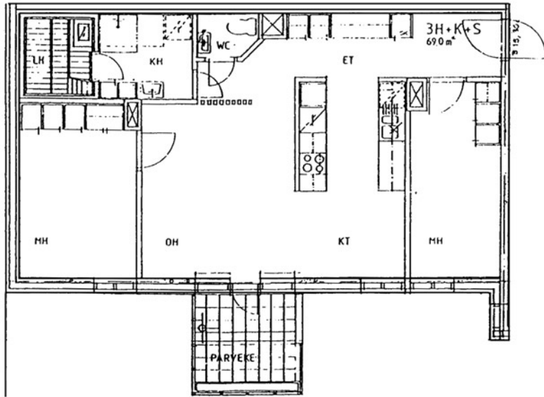
Saimaankatu 58 B A 11 / pohjakuva Ei mittakaavassa
