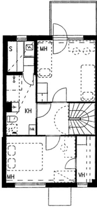
Kustaankatu 1 C 8 / pohjakuva 2. kerros Ei mittakaavassa
