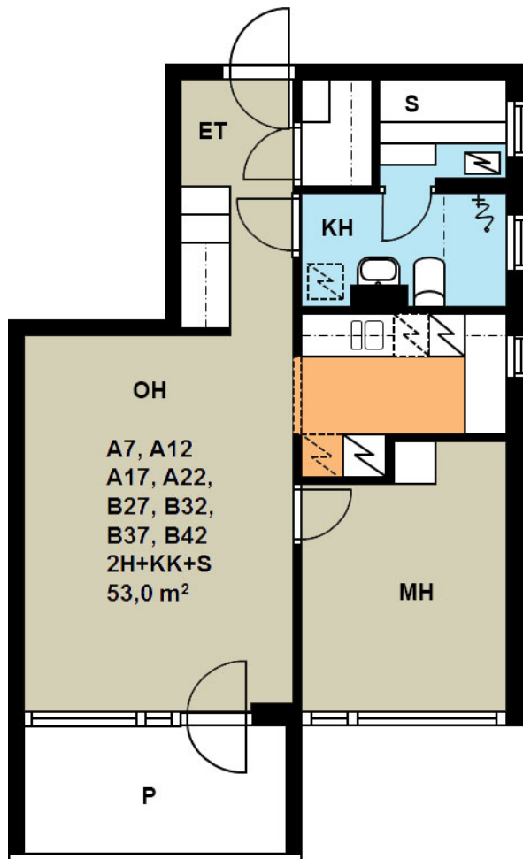
Numersinkatu 3 B 27 / Pohjakuva Ei mittakaavassa
