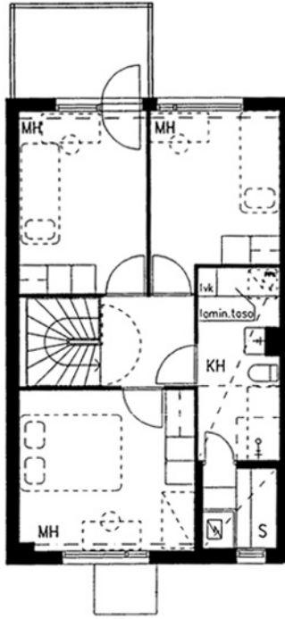
Kustaankatu 1 C 5 / pohjakuva 2. kerros Ei mittakaavassa
