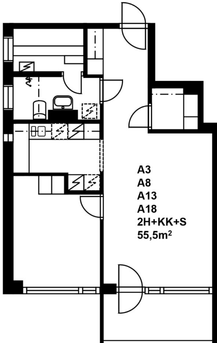
Numersinkatu 3 A 18 / Pohjakuva Ei mittakaavassa
