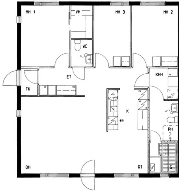
Lehtikummuntie 8 C 5 / pohjakuva Ei mittakaavassa
