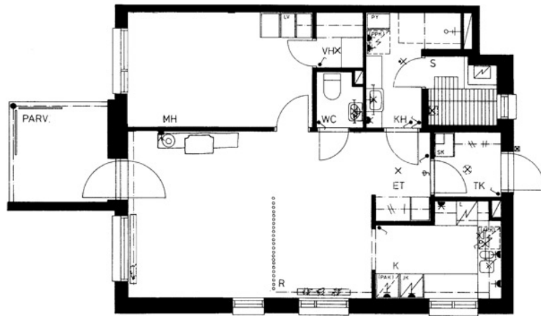
Snellmanintie 9 C 20 / pohjakuva Not in scale
