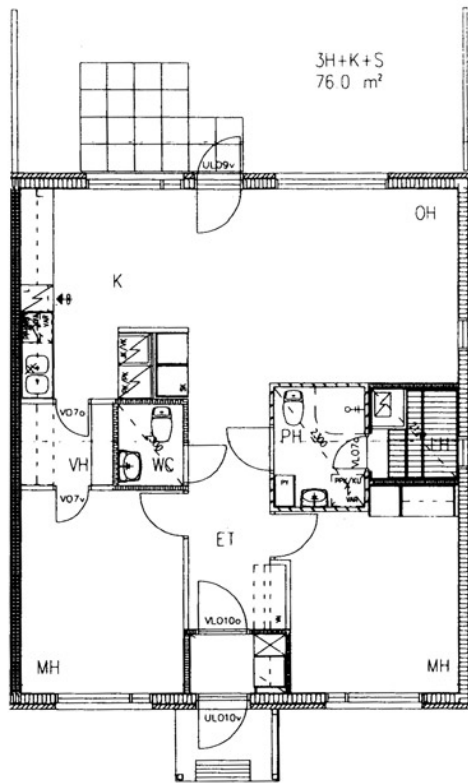
Penttilänkatu 20 C 16 / pohjakuva Not in scale
