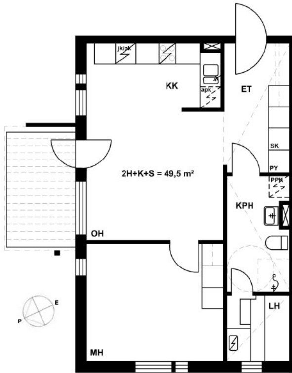
Läntinen Kanavatie 27 As 8 / Pohjakuva Ei mittakaavassa
