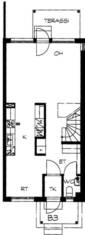
Lyhtykuja 1-3 B 3 / pohjakuva 1.kerros Ei mittakaavassa
