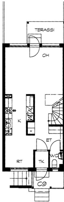
Lyhtykuja 1-3 C 9 / pohjakuva 1.kerros Ei mittakaavassa
