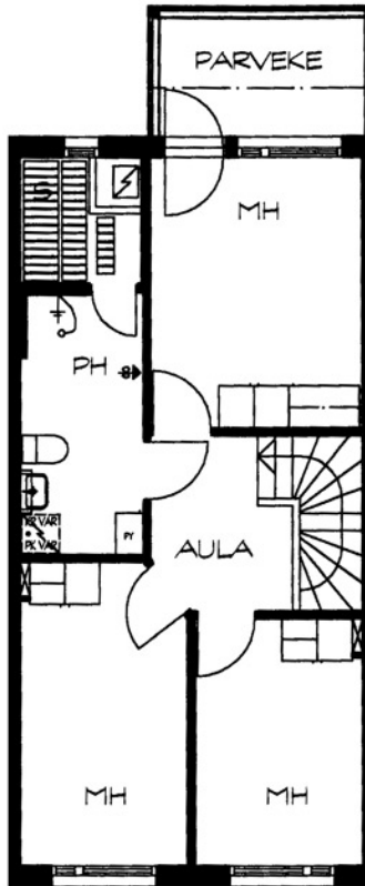
Lyhtykuja 1-3 C 9 / pohjakuva 2.kerros Ei mittakaavassa
