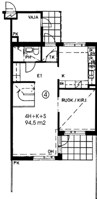
Orminkuja 5 A 4 / pohjakuva 1. kerros Ei mittakaavassa
