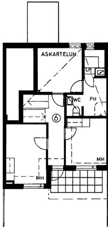
Orminkuja 5 B 6 / pohjakuva 1. kerros Ei mittakaavassa
