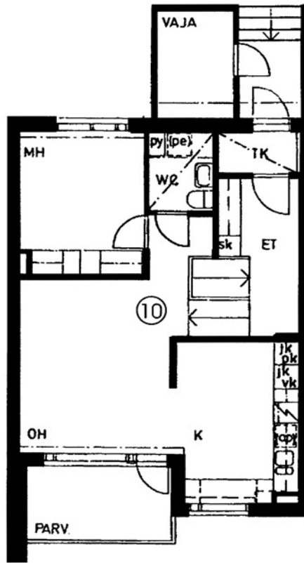
Orminkuja 5 C 10 / pohjakuva 2. kerros Not in scale
