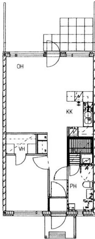
Rälssimiehentie 8-10 V / pohjakuva Ei mittakaavassa
