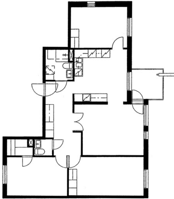
Ounasvaarantie 7 D 53 / pohjakuva Ei mittakaavassa
