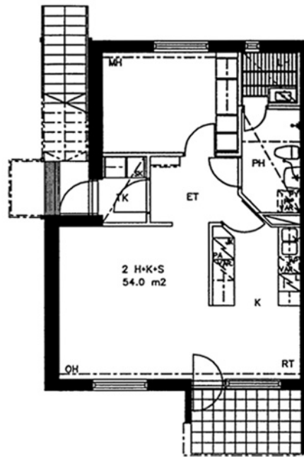
Huvipurentie 1 C 15 / pohjakuva Ei mittakaavassa
