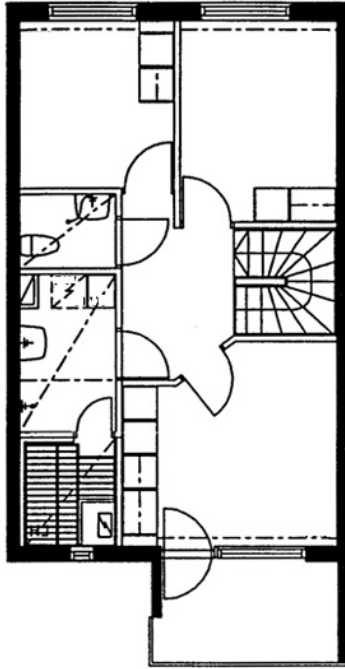
Huvipurentie 1 C 18 / pohjakuva 2. kerros Ei mittakaavassa
