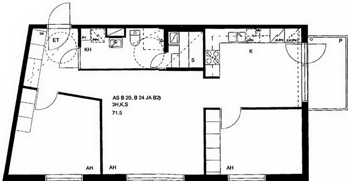
Lähtetiläntie 2 B 20 / Pohjakuva Ei mittakaavassa
