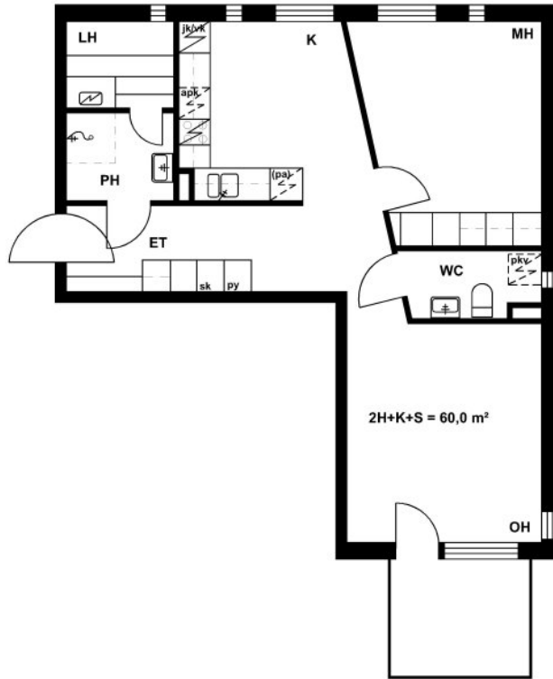
Takaniityntie 3 C 20 / Pohjakuva Ei mittakaavassa
