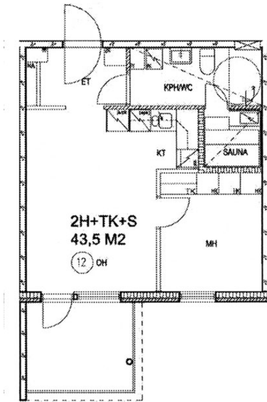
Dunckerinkatu 4 B 31 / pohjakuva Ei mittakaavassa
